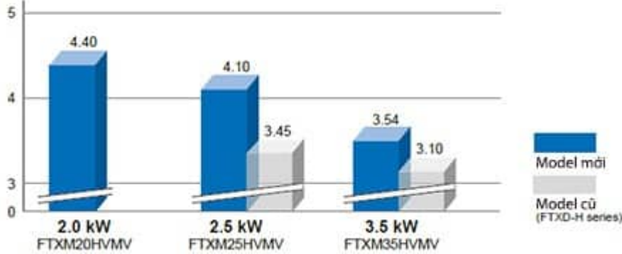
COP danh định (W/W) trong vận hành làm lạnh
